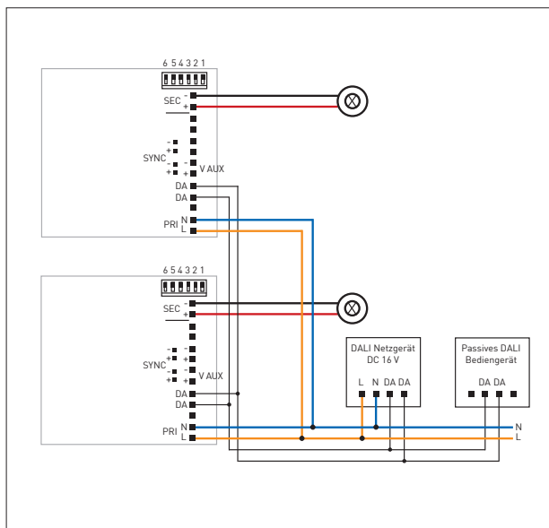
Schaltbild: DALI-Netzgerät und passiven Bediengerät
