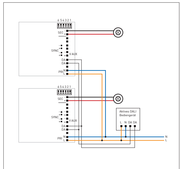
Schaltbild: DALI-Potentiometer mit integriertem Netzteil
