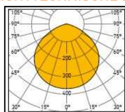
120° Abstrahlwinkel
